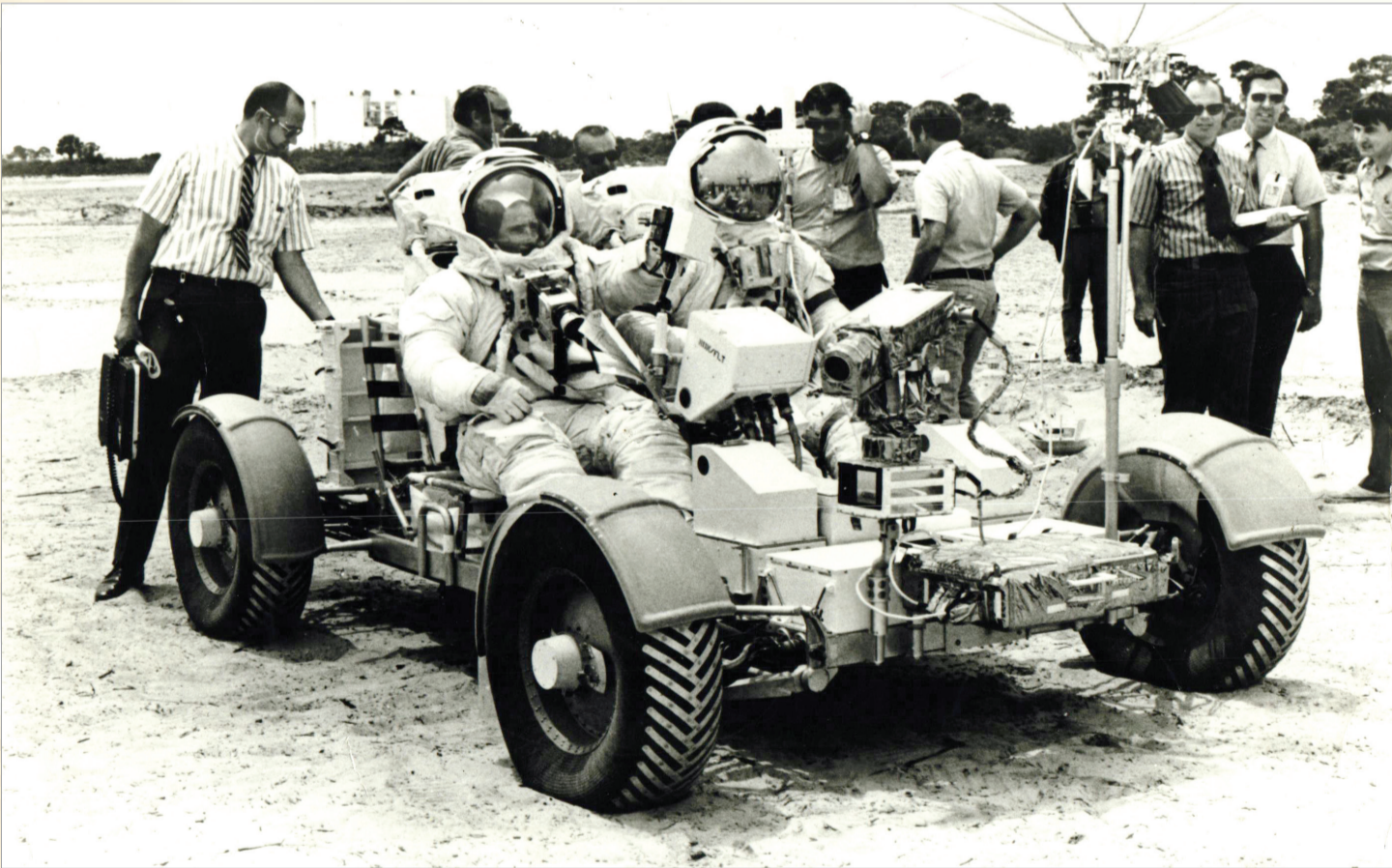
برنامج طيران الفضاء (ابولو) والذي قامت به (ناسا) بالولايات المتحدة الأمريكية وكان يهدف لتوصيل وهبوط البشر على سطح القمر
